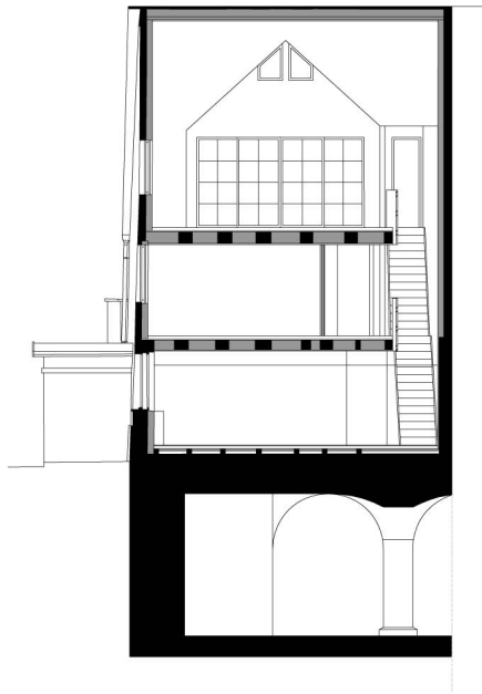
SCHNITT A-A
