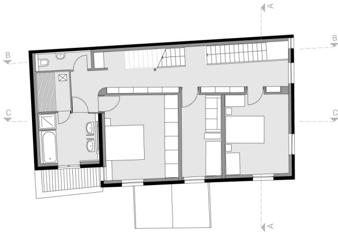
OBERGESCHOSS
